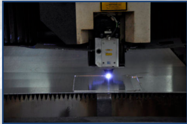
Laserschneiden
